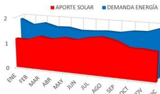
Figura 112: Variación anual de la demanda de energía para ACS y el aporte solar
