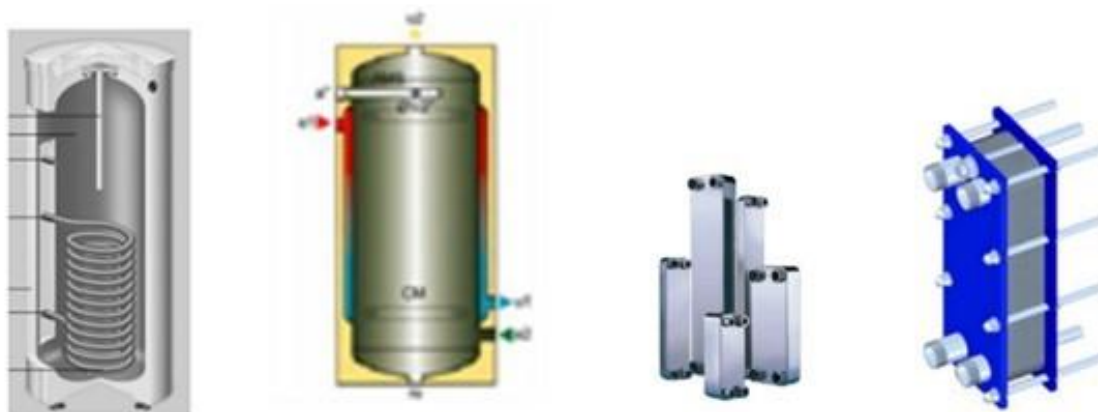
Figura 30: Diversos tipos de intercambiador: incorporados y externos
