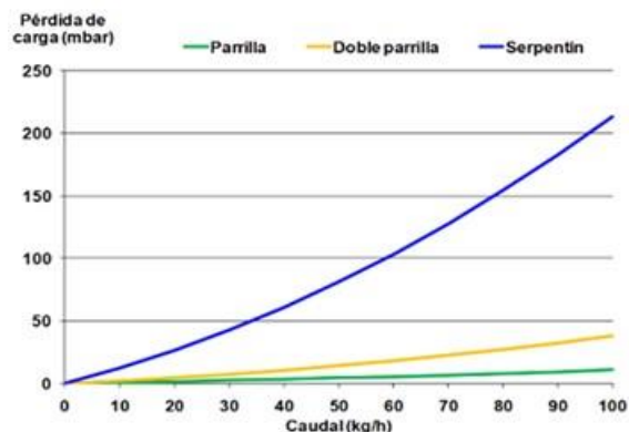
Figura 26: Pérdida de carga de tres tipos de absorbedor
