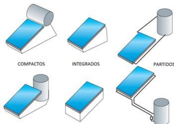
Figura 9: Formas de acoplamiento
