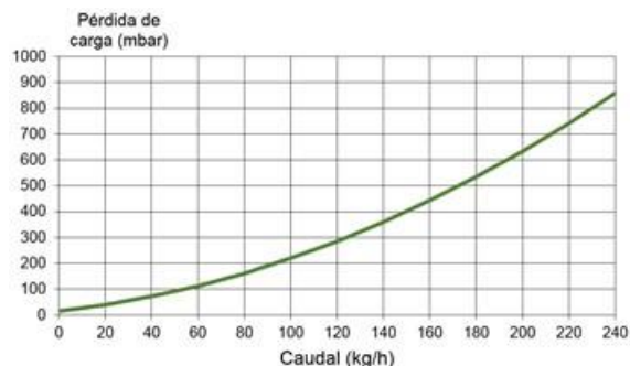
Figura 60: Ejemplo de pérdida de carga de un captador en función del caudal másico
