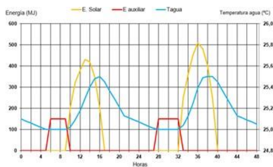
Figura 109: Evolución temporal de temperaturas del agua del vaso, de la energía solar y la auxiliar
