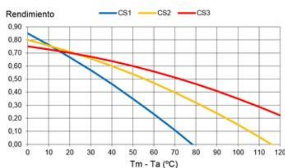
Figura 25: Rendimiento de tres tipos de captador solar
