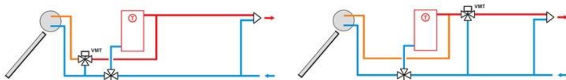
Figura 48: Esquema de conexionado en paralelo con válvula de tres vías manual para conmutación y válvula mezcladora para el sistema solar (izq.) o para sistemas solar y auxiliar (der.)
