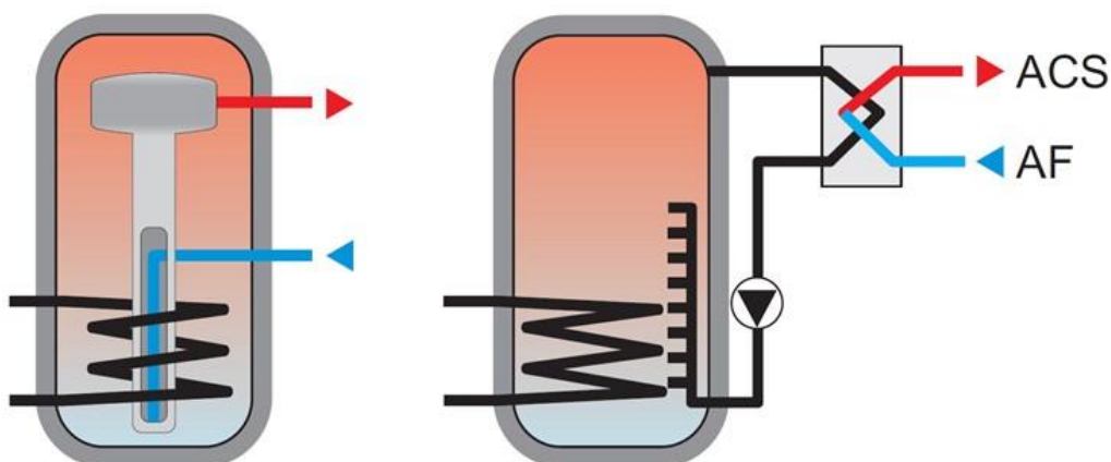
Figura 118: Ejemplos de acumuladores para ACS y calefacción con elementos estratificadores
