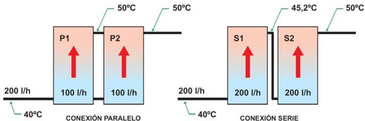
Figura 59: Ejemplos de conexionado en paralelo y en serie de dos captadores solares
