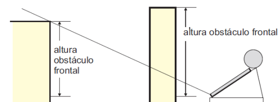
Figura 36: Obstáculos frontales y laterales que pueden producir sombras.
