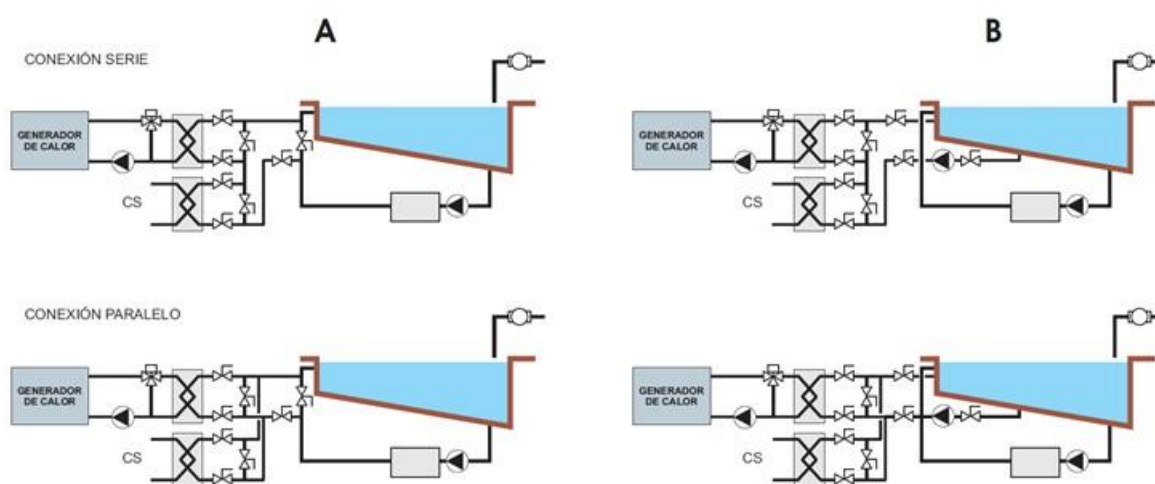
Figura 107: Opciones de conexionado de los intercambiadores de calentamiento, solar y convencional, en serie o en paralelo, para los dos casos de utilizar circuito de depuración (A) o circuito independiente (B)
