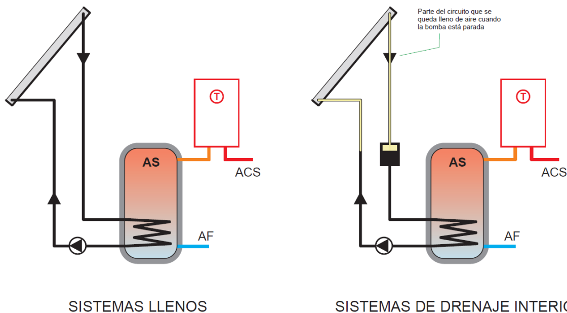
Figura 8: Tipos de circuitos primario según su contenido de líquido
