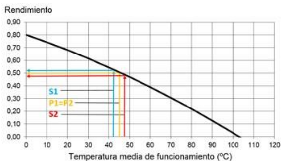
Figura 61: Rendimientos del captador y puntos de trabajo en función de su temperatura
