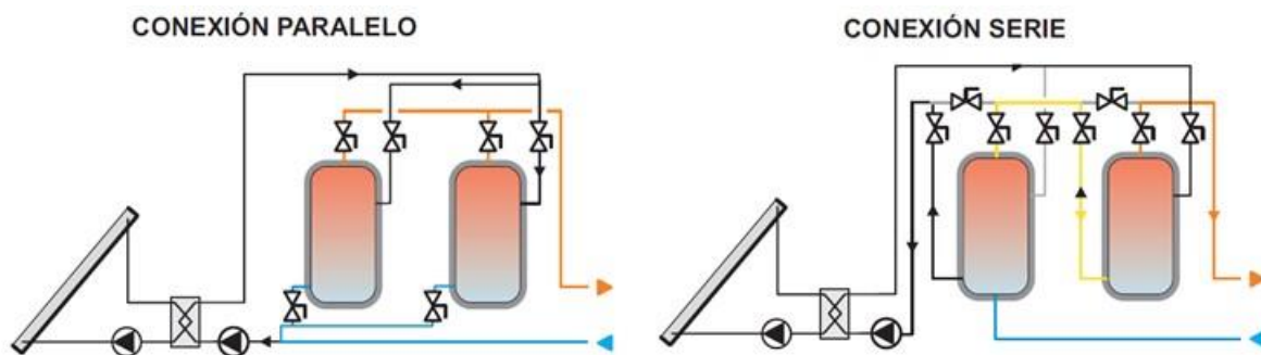
Figura 67: Conexión de dos acumuladores, calentados por intercambiador externo, en paralelo y en serie
